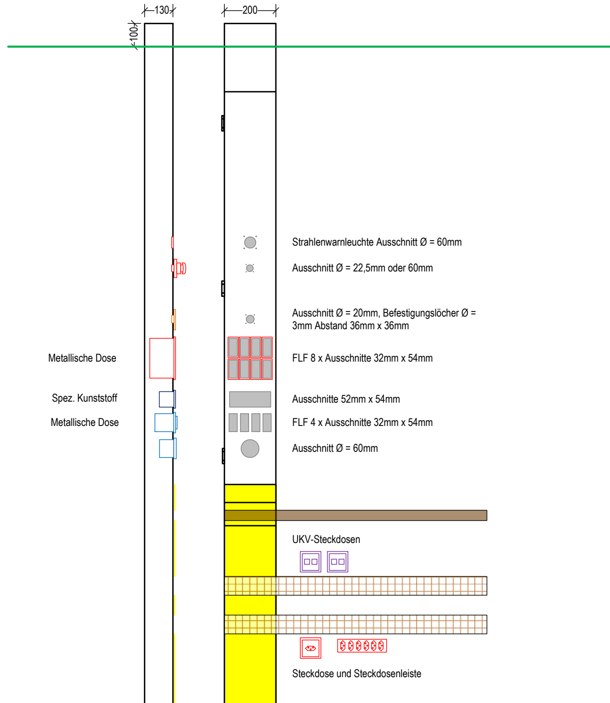
Abbildung 3, Konsole Hohldecke
