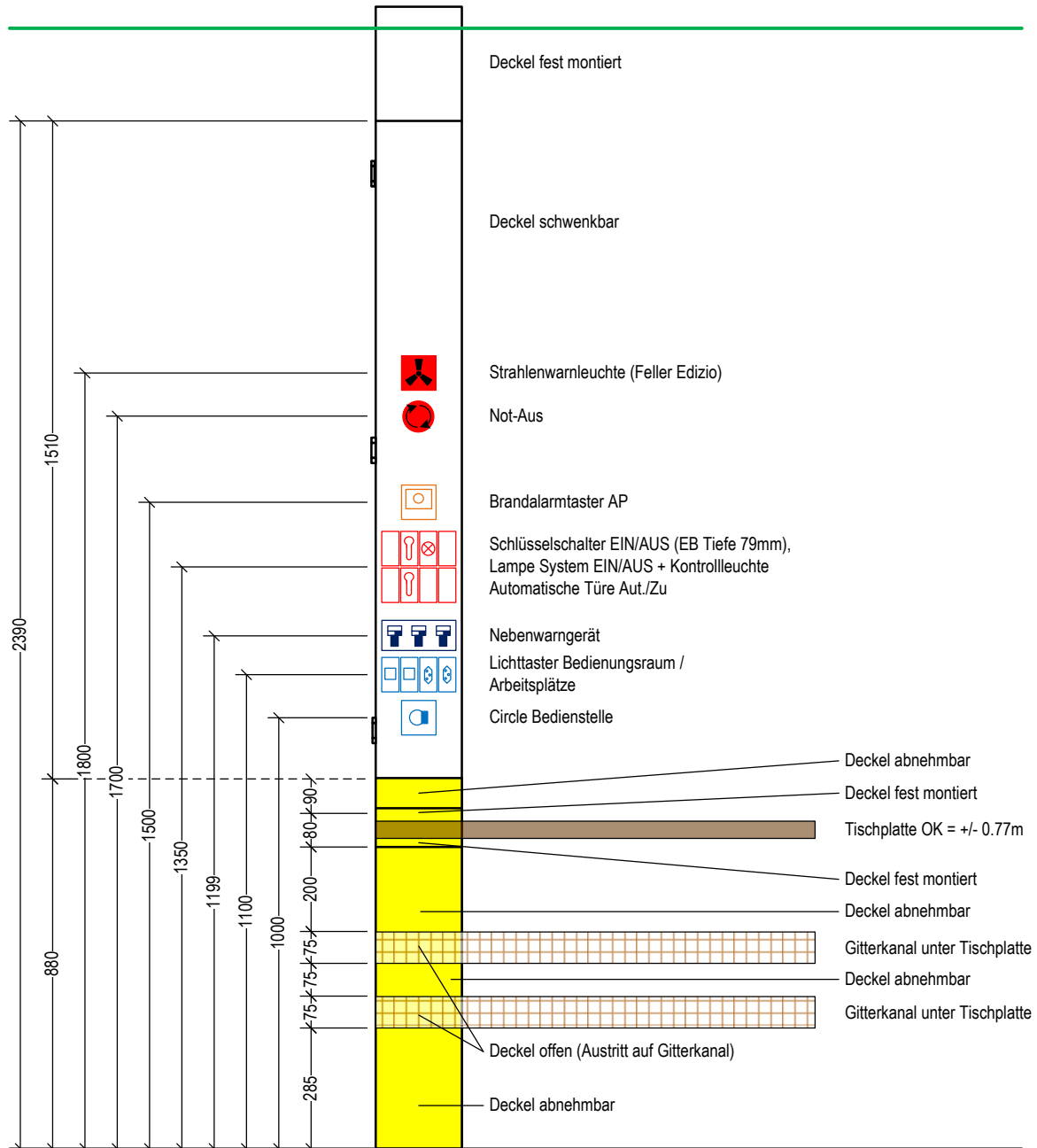
Abbildung 2, Konsole Festdecke
