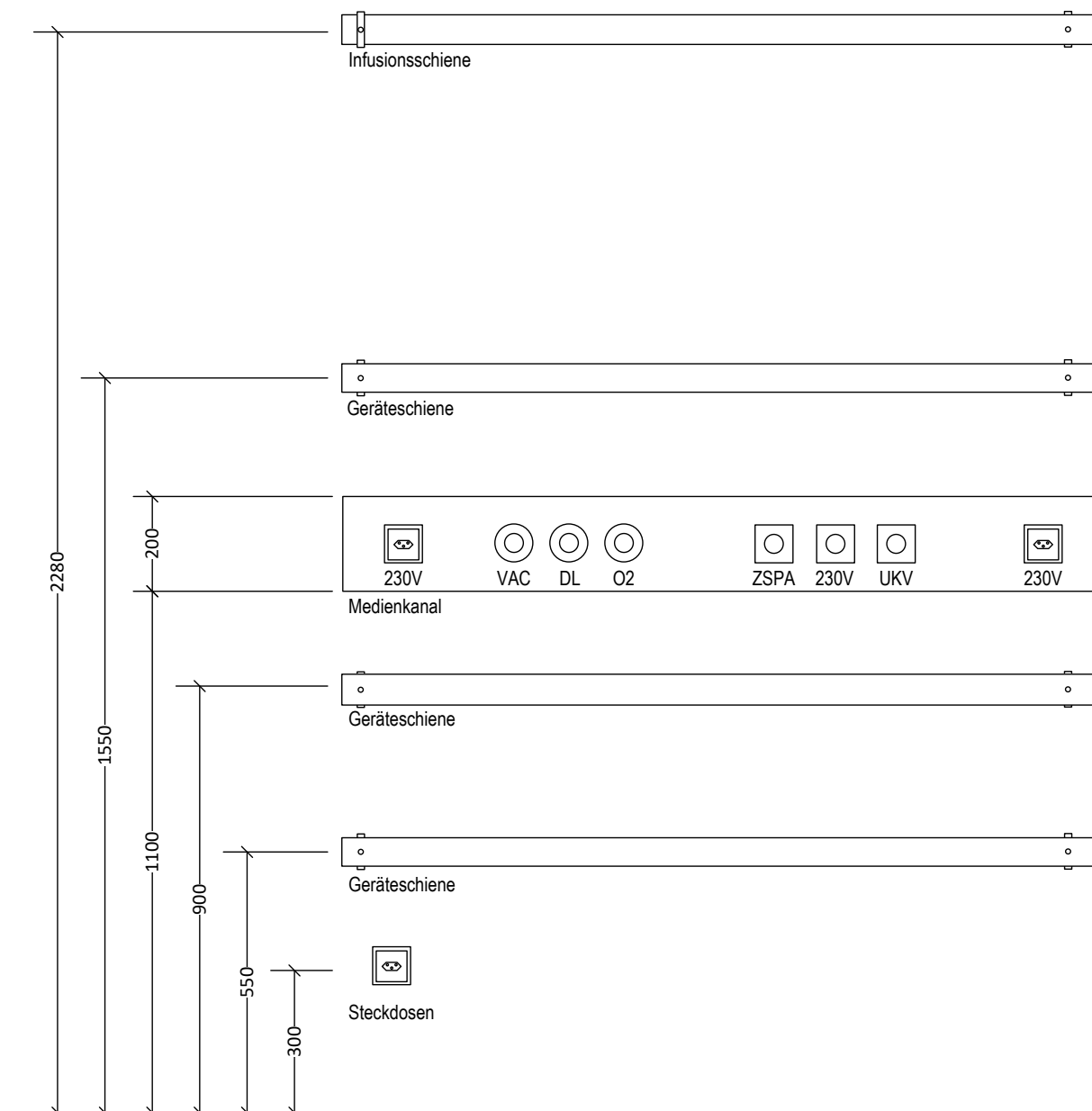
Abbildung 4, Geräteschienen Patientenzimmer
