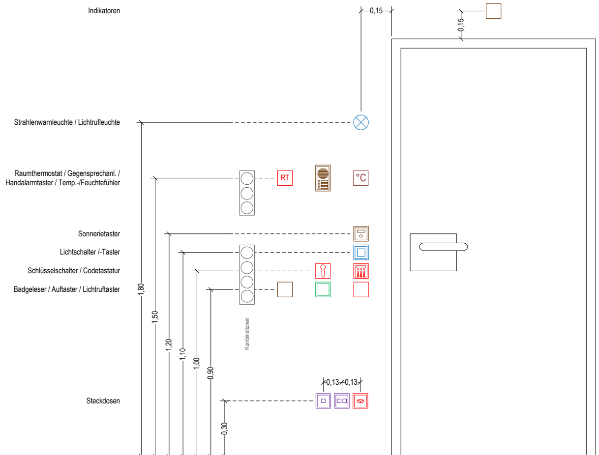
Abbildung 1, Anordnung Türen
